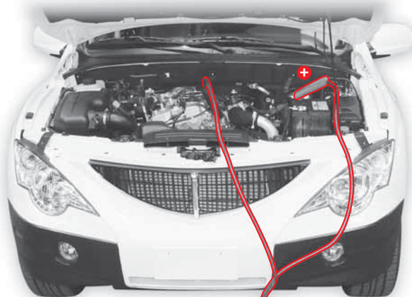
Разряженный аккумулятор
